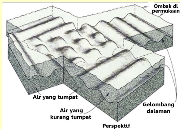
Rajah 16: Gelombang dalaman yang berlaku di interfasa antara dua lapisan air yang mempunyai ketumpatan yang berbeza. Satu mempunyai ketumpatan yang tinggi (lapisan bawah), yang satu lagi mempunyai ketumpatan yang lebih rendah (lapisan atas). ( Oceanography , Gross, ms.204)
