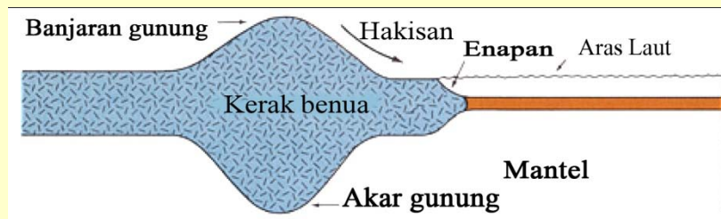
Rajah 9: Satu lagi ilustrasi yang menunjukkan bagaimana gunung mempunyai bentuk seperti pancang kerana akarnya yang dalam ( Earth Science , Tarbuck dan Lutgens, ms. 158.)
