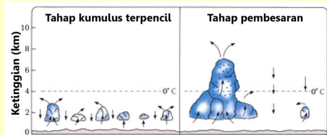
Rajah 19: (A) Kepingan awan-awan kecil yang terasing (awan kumulus). (B) Apabila awan-awan kecil ini bercantum, arus menaik di dalam awan yang lebih besar itu meningkat, dan menyebabkan awan itu bertimbun. Titisan air ditunjukkan dengan . ( The Atmosphere , Anthes dan lain-lain, ms. 269.)
