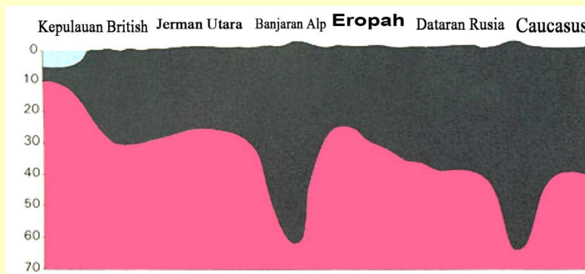
Rajah 8: Keratan skema. Gunung, seperti pancang, mempunyai akar yang dalam yang terbenam di dalam bumi ( Anatomy of the Earth , Cailleux, ms. 220.)
