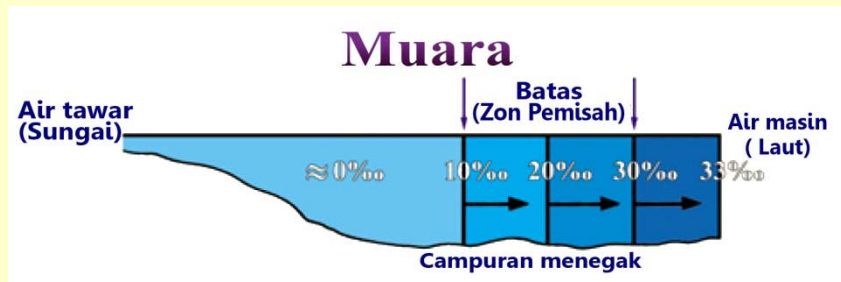
Rajah 14: Keratan rentas menunjukkan kemasinan (bahagian per ribu ‰) di muara. Kita boleh melihat di sini, batas (zon pemisah) di antara air tawar dengan air masin. ( Introductory Oceanography , Thurman, ms. 301, dengan sedikit penambahan.)
