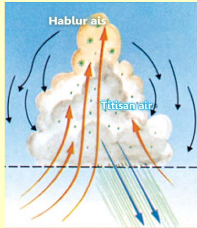
Rajah 20: Awan kumulonimbus. Setelah awan menimbun ke atas, hujan turun darinya. ( Weather and Climate , Bodin, ms.123.)
