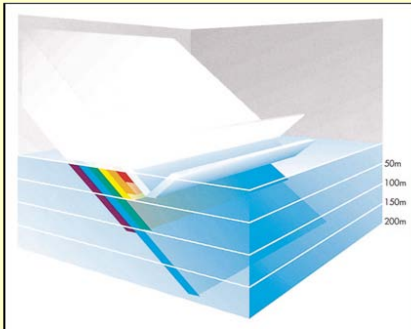
Rajah 15: Antara 3 hingga 30 peratus cahaya matahari dipantul pada permukaan laut. Setelah itu, hampir kesemua warna di dalam spektrum cahaya diserap satu per satu pada kedalaman 200 meter pertama, kecuali cahaya biru. ( Oceans , Elder dan Pernetta, ms. 27.)
