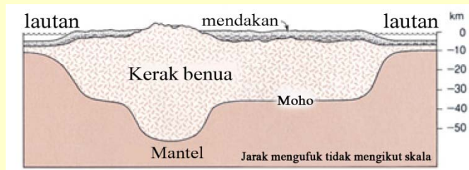
Rajah 7: Gunung-ganang mempunyai akar yang dalam di bawah permukaan bumi. ( Earth , Press dan Siever, ms. 413.)
