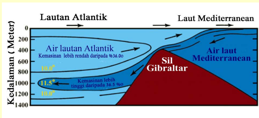
Rajah 13: Air dari Laut Mediterranean memasuki Lautan Atlantik menyeberangi sil Gibraltar dengan ciri-cirinya yang tersendiri; lebih panas, lebih masin dan kurang tumpat, kerana benteng yang memisahkan kedua-duanya. Suhu di dalam darjah Celsius(°C). ( Marine Geology , Kuenen, ms.43, dengan sedikit penambahan.)
